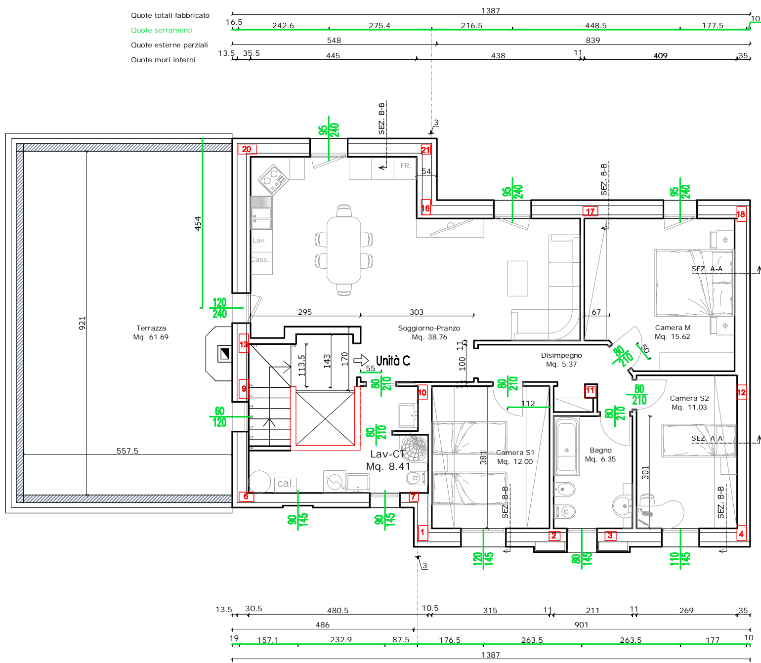
Pianta Piano Secondo - Unità C - Scala 1:100
