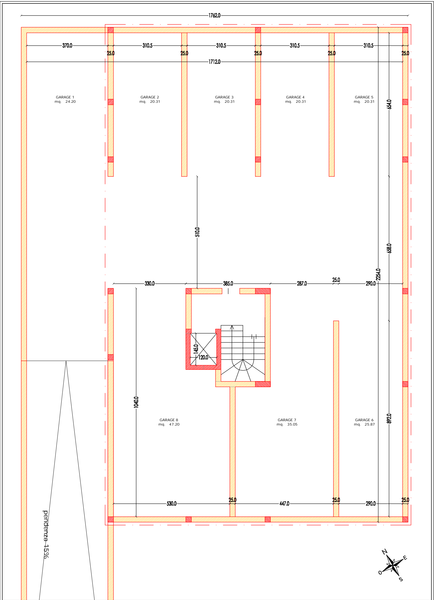
PIANO INTERRATO - Scala 1:100
