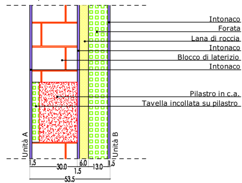
Vista su pilastro in Pianta
