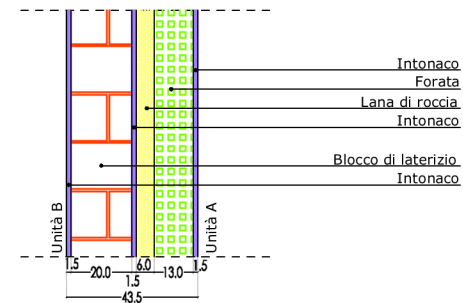
Tra unità A e B
