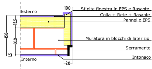
Particolare Pianta su Finestra
