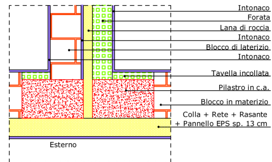
Vista su Pilastro in Pianta
