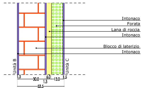
Tra unità B e C
